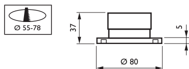
Produkt na ilustracji: BBW300 Wszystkie wymiary są podane w mm
