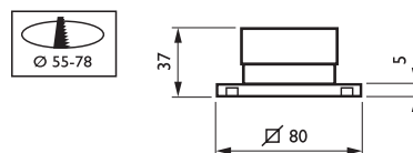
Produkt na ilustracji: BBW301 Wszystkie wymiary są podane w mm
